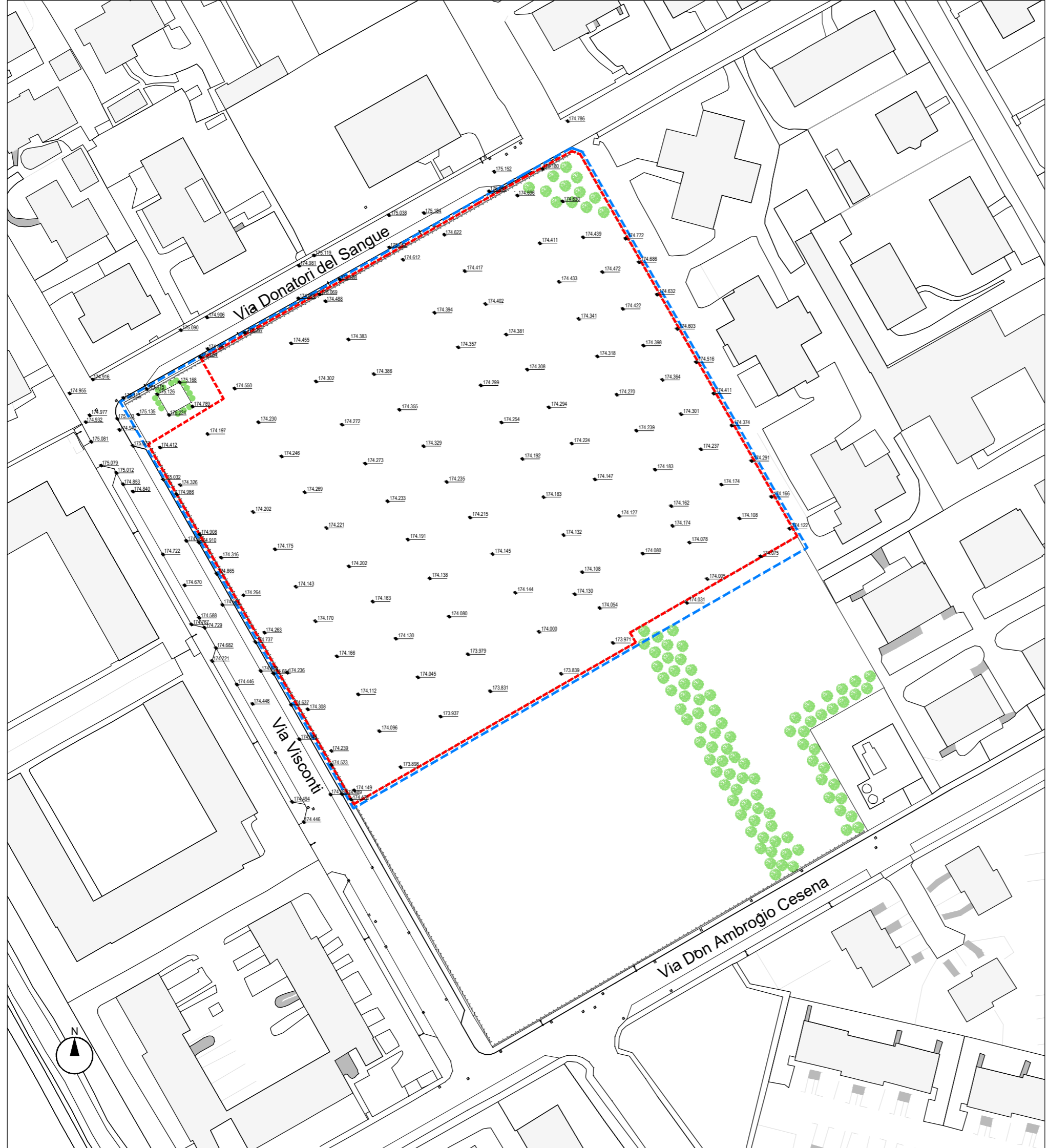
PLANIMETRIA GENERALE_STATO DI FATTO E PERIMETRAZIONE SU BASE RILIEVO STRUMENTALE
